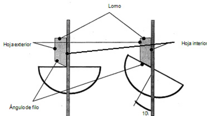
Figura 3 - Lectura del ángulo de filo
